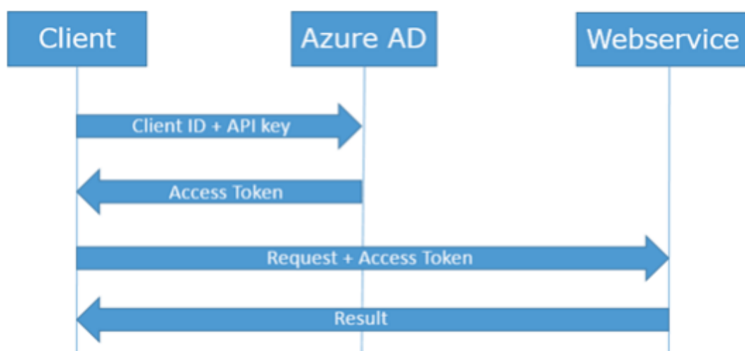
Figuur 1: authenticatieflow
